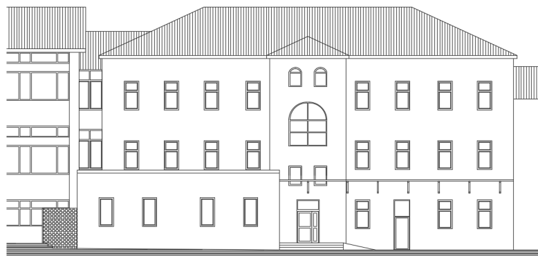
Slika 5: Zahodna fasada
